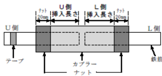
図2 機械式継手試験体
